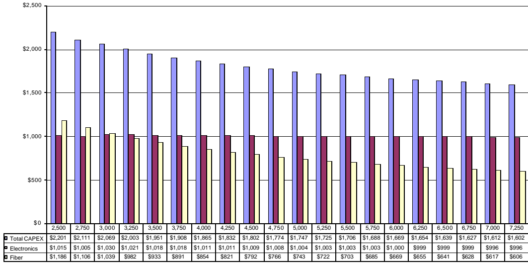
CAPEX per HH vs No HH (GigE)
